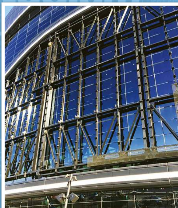
4200 Type AAF soutiennent l'écran de 83 mètres
