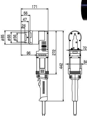
GHC-241EZ GHC-242EZ
