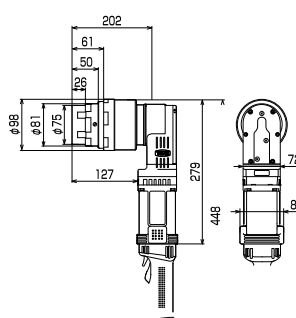
GVC-301 GVC-302
