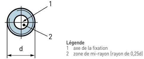
5.0-25 - Zone de mi-rayon pour la détermination de la dureté
