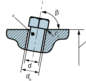
5.0-23 - Dispositif d'essai de solidité de la tête
