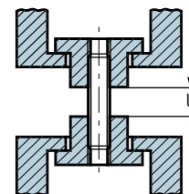
Figure d - Exemple de dispositif d'essai pour les tiges filetées
